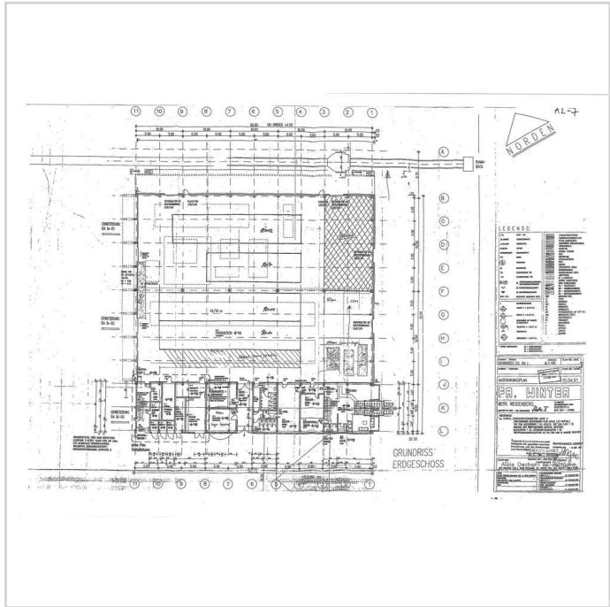
22 Grundriss Erdgeschoß
